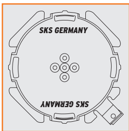
11695 Bajonettaufnahme/Bayonet mount
