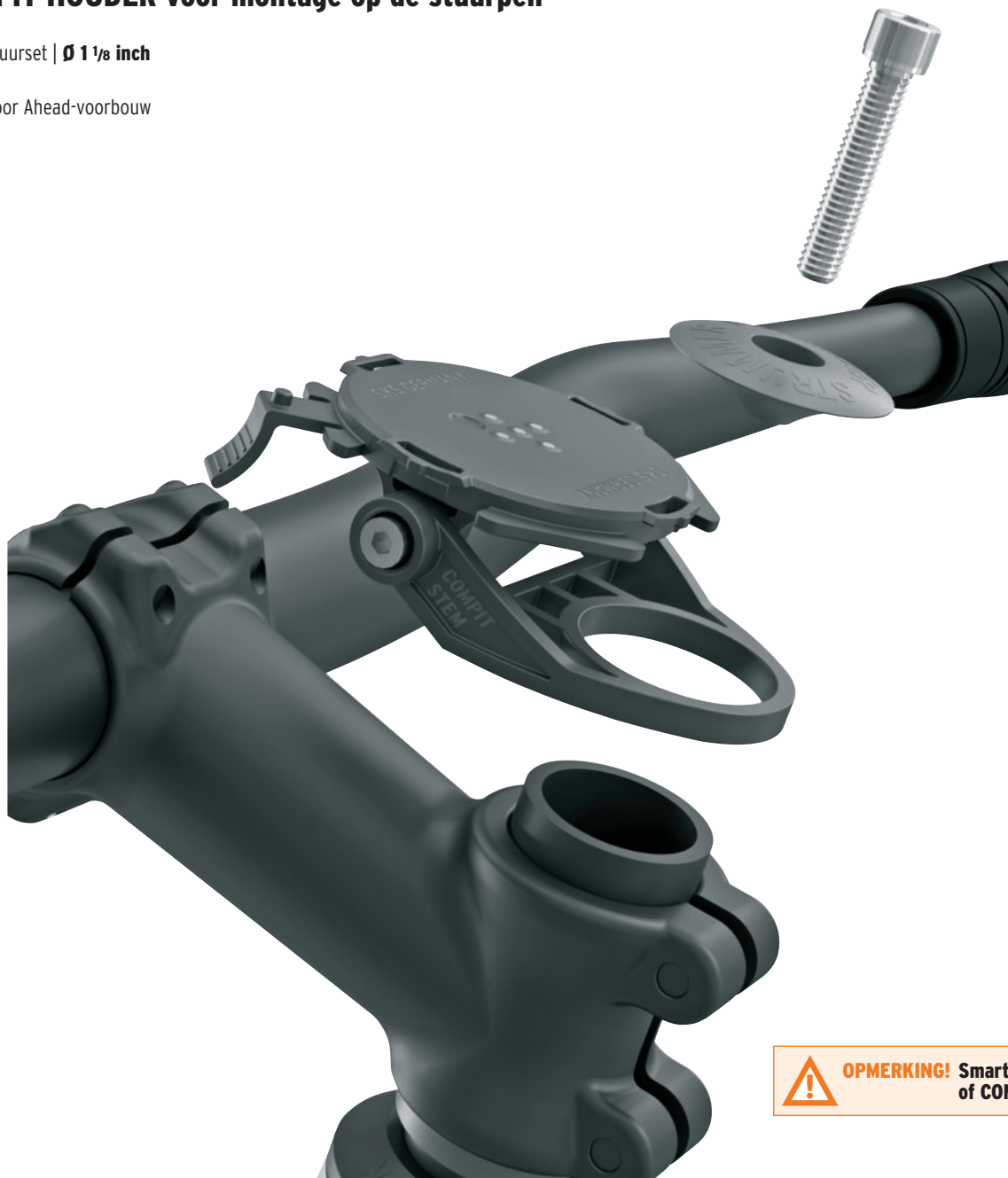
Alternatieve montage 1
