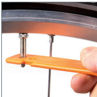
Schlüssel für das innere SV-Ventil
